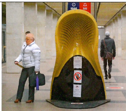
Dieses Gerät in der Botanitscheski-Sad-Station in der Moskauer U-Bahn dämpft durch Interferenz die Umgebungsgeräusche
